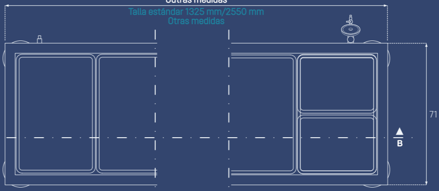
Planta Plano de planta
