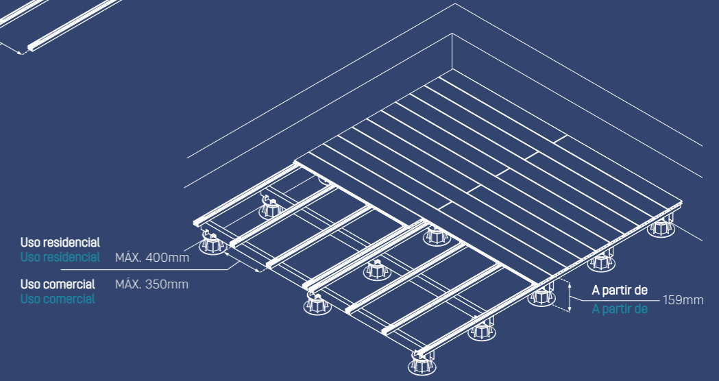
INSTALAÇÃO ELEVADA INSTALACIÓN ELEVADA
