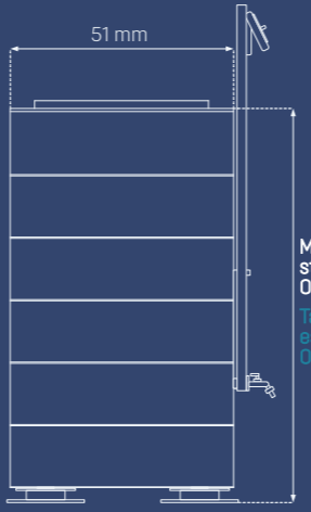
Alçado lateral Alzado lateral
