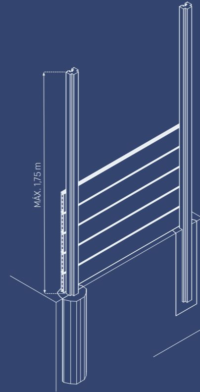
FIXAÇÃO DIRETA NO SOLO COM MACIÇO DE BETÃO FIJACIÓN DIRECTA EN EL SUELO COM MACIZADO DE HORMIGÓN
