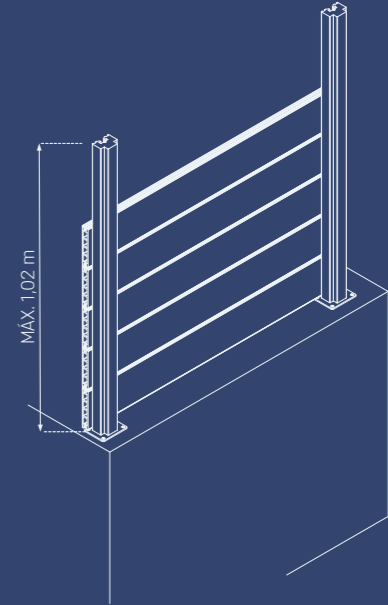
FIXAÇÃO COM FIXADORES EM BASE DE BETÃO FIJACIÓN CON FIJADORES EN BASE DE HORMIGÓN
