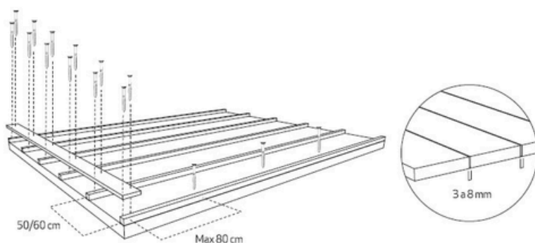
DESENHO TÉCNICO
